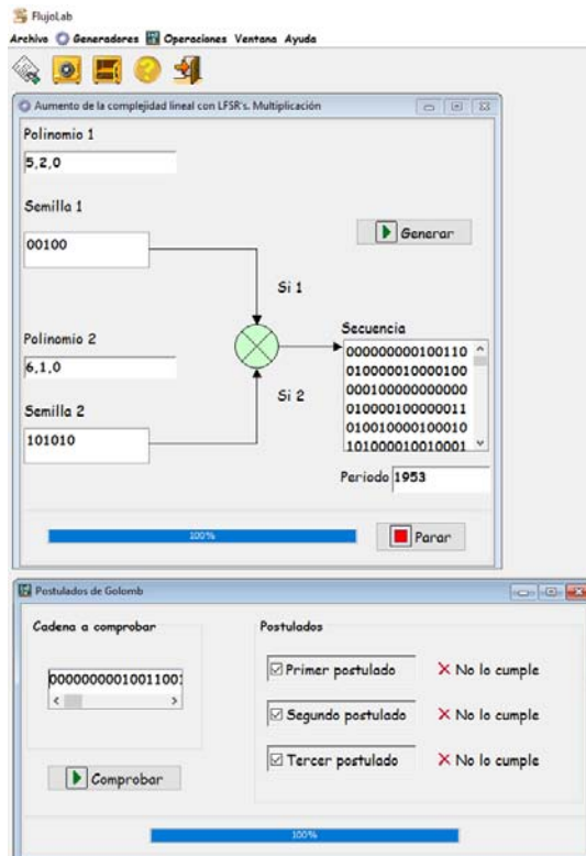
Figura 18. Secuencia multiplicación con dos polinomios primitivos (5,2,0) y (6,1,0).
